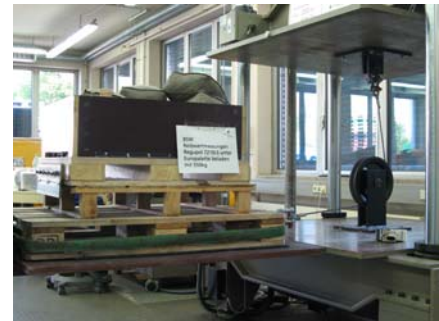
Zugkraftmessung mit Kufen parallel zur Zugrichtung
